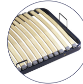
3 poignées soudées maintiennent le matelas en place
